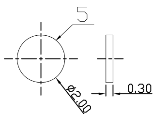
MMCX公頭(公PIN)-墊片
