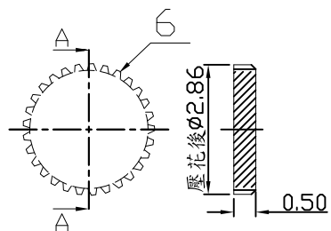
A-A剖視圖
