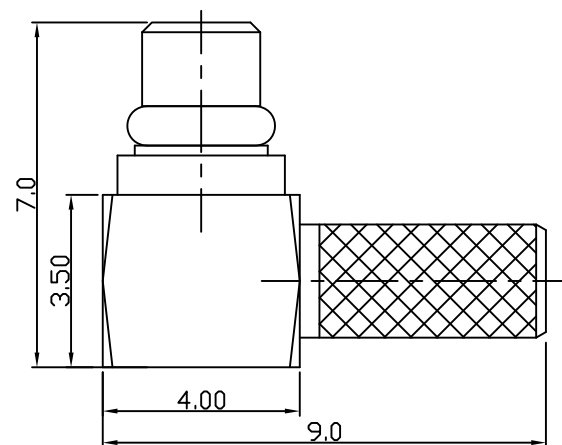
MMCX公頭(公PIN)-組件1
