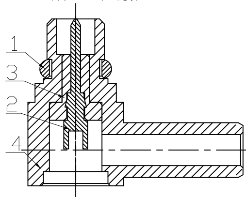
MMCX公頭(公PIN)-後套
