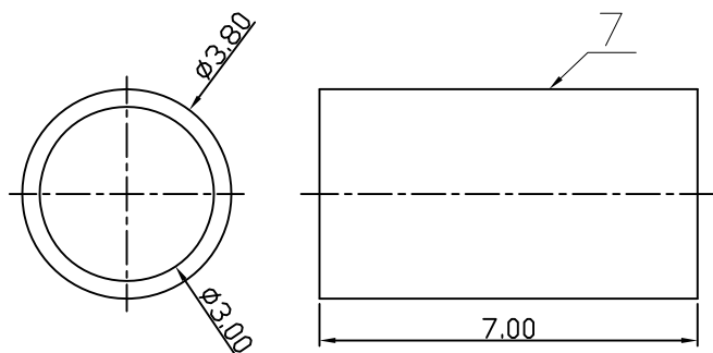
MMCX公頭(公PIN)-後套
