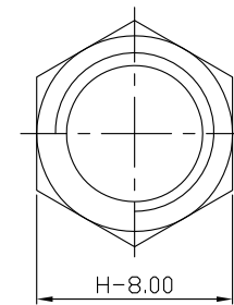
螺母 CD013932032-5
