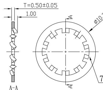
銅墊圈 CD013922002-4
