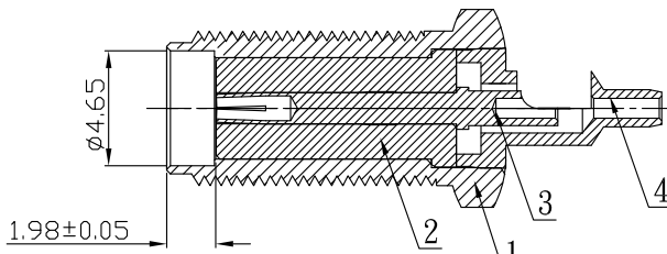
組件 CD015942018-6
