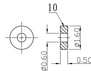
SCALE 4:1 CD013942022-5
