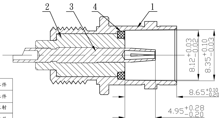
A-A' 剖視圖
