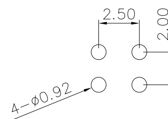
PCB LAYOUT(SCALE:4X)
