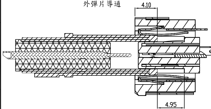
內彈片導通
