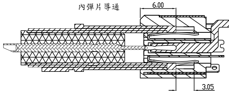
母端子導通
